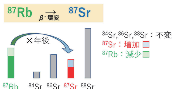
図 1. Rb の放射壊変と Sr 安定同位体の変化
