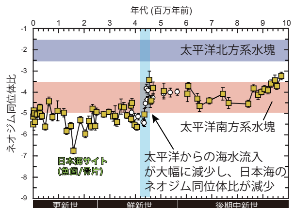
図 4. 日本海堆積物中の魚歯・骨片化石のネオジム同位体比の過去 1000 万年間の変動。同時期の太平洋北方系水塊と南方系水塊のネオジム同位体比も合わせて示した。450 万年前に日本海のネオジム同位体比の急激な減少が見られる。
