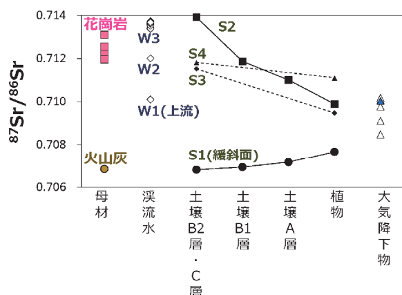
図 2. 森林の各種試料の Sr 同位体比。土壌は層別別に分析した。
