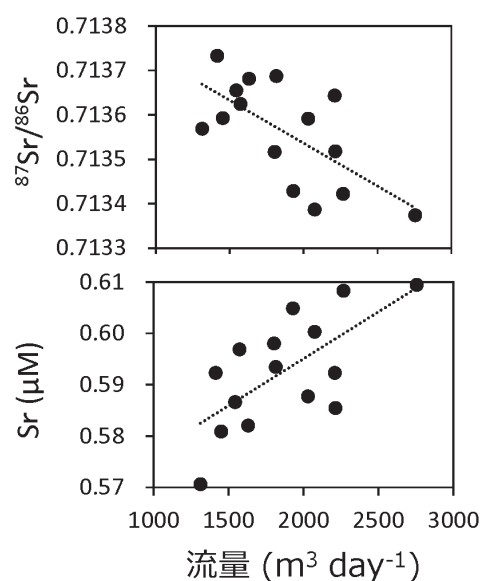
図 4. 渓流水の流量と Sr 同位体比や Sr 濃度の関係
