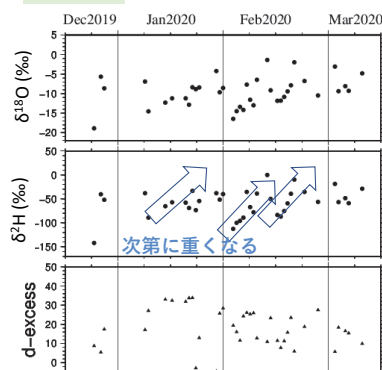
図 3. 弘前における第 1 冬季（2019 年 12 月～2020 年 3 月）の降水の酸素同位体比、水素同位体比、d-excess。
