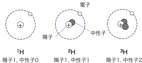
図2. 水素の同位体の例 原子番号1の水素には陽子1個と中性子0個を持つ安定同位体 ^1\text{H} 、陽子1個と中性子1個を持つ安定同位体 ^2\text{H} （重水素、デューテリウム、Dとも書く）、陽子1個と中性子2個を持つ放射性同位体 ^3\text{H} （三重水素、トリチウム、Tとも書く）があります。
